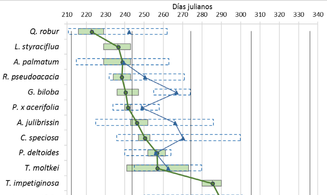
Figura 1. Secuencia fenológica de las especies forestales de agosto a noviembre. La fecha media de comienzo de brotación para cada especie en los distintos períodos está indicada por las líneas punteada (2015-2017) y llena (1947-1956). Las líneas negras verticales indican el comienzo de cada mes de agosto a noviembre. Las barras horizontales indican las fechas extremas de comienzo de fase para los períodos 2015-2017 y 1947-1956 (verde y azul punteada, respectivamente), para cada especie. L. styraciflua y T. impetiginosa no tienen registros fenológicos durante el período 1947-1956.
